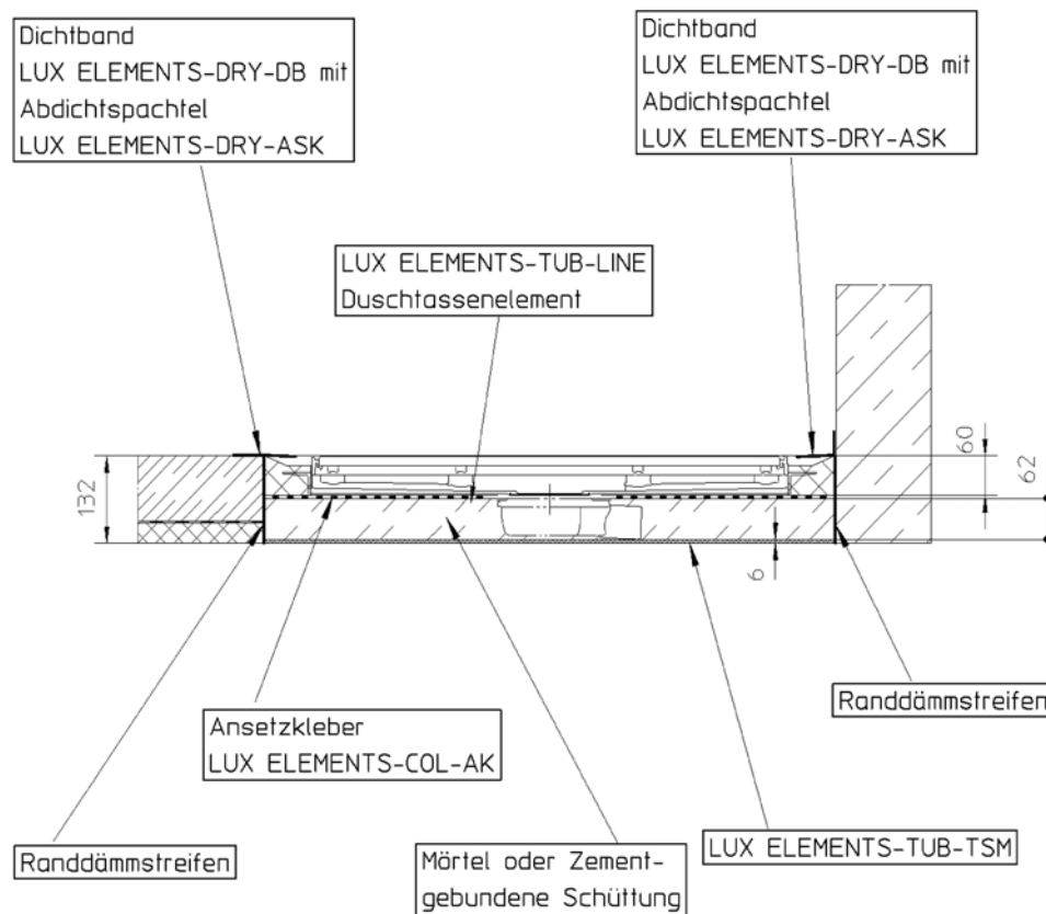
Abbildung 1: LUX ELEMENTS-TUB-LINE mit waagerechtem Ablauf und Estrich
