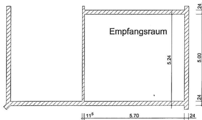
Grundriss Erdgeschoss
