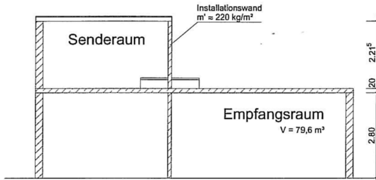
Schnitt
