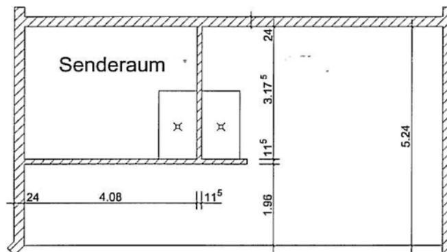
Grundriss Obergeschoss
