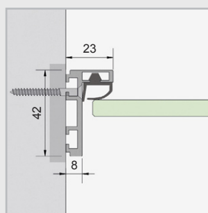
Kozijnprofiel
