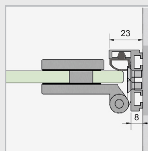
Kozijnprofiel deurscharnier
