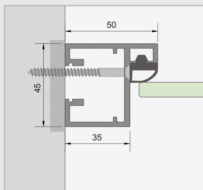
Kozijnprofiel
