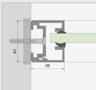
Wandprofiel
