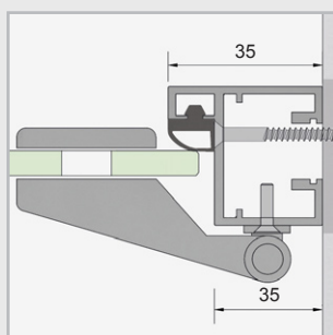
Kozijnprofiel deurscharnier
