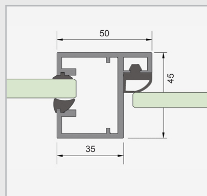
Kozijnprofiel, aansluiting wandprofiel
