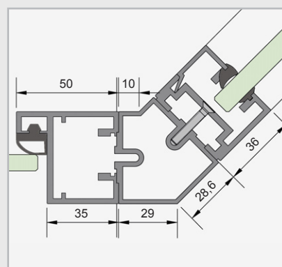
Kozijnprofiel met hoekprofiel 135° + wandprofiel
