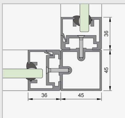
2x wandprofiel met hoekprofiel 90°
