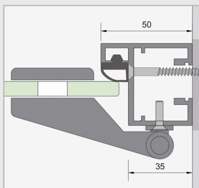
Kozijnprofiel deurscharnier
