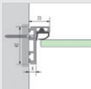
Kozijnprofiel, wandaansluiting
