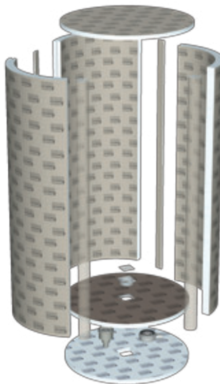
Bouwpakket ronde douche – RELAX-RD
