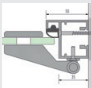
Kozijnprofiel deurscharnier, wandaansluiting
