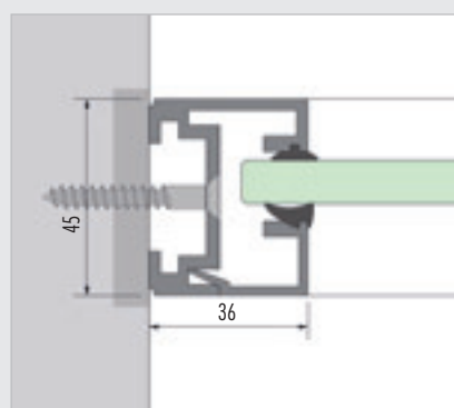
Wandprofiel, wandaansluiting
