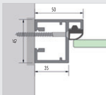
Kozijnprofiel, wandaansluiting
