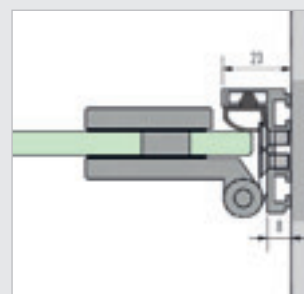
Kozijnprofiel deurscharnier, wandaansluiting
