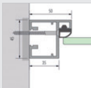
Kozijnprofiel, wandaansluiting
