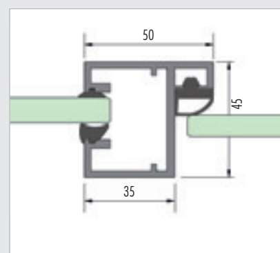
Kozijnprofiel, aansluiting wandprofiel
