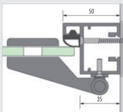
Kozijnprofiel deurscharnier, wandaansluiting
