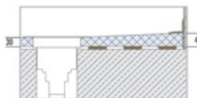
Afvoer verticaal zonder onderbouwelement
