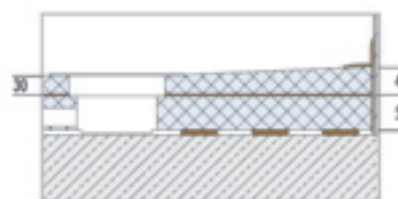
Afvoer horizontaal met onderbouwelement
