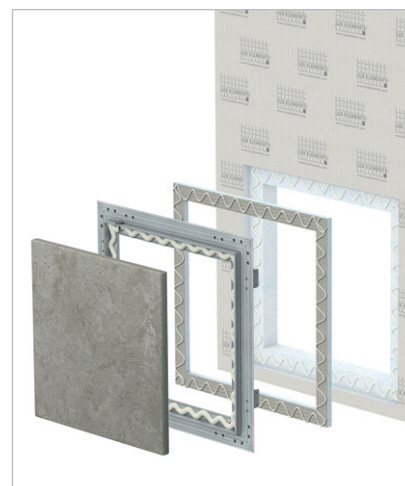
Gebruik bij natuursteen: zonder frontplaat / vulstukken onder frame
