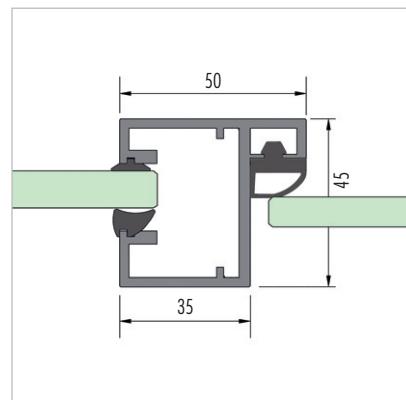
3 Kozijnprofiel, aansluiting wandprofiel
