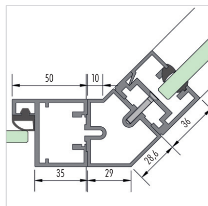
6 Kozijnprofiel met hoekprofiel 135° + wandprofiel
