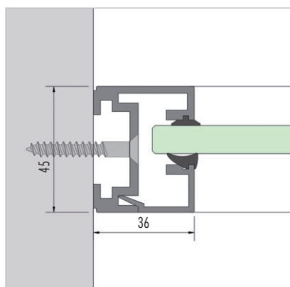
4 Wandprofiel, wandaansluiting
