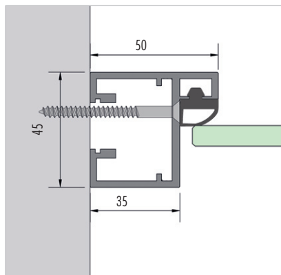
1 Kozijnprofiel, wandaansluiting
