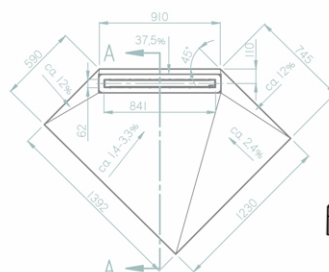
Receveur de douche avec écoulement en ligne TUB-LINE PLUS Fabrication sur mesure → à partir de la page 34
