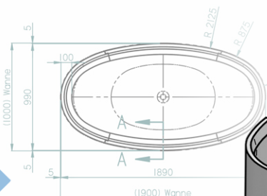
Habillage de baignoire TOP PLUS Fabrication sur mesure → page 72
