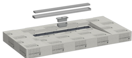
Plan vasque LAVADO-FLOAT Produit standard
