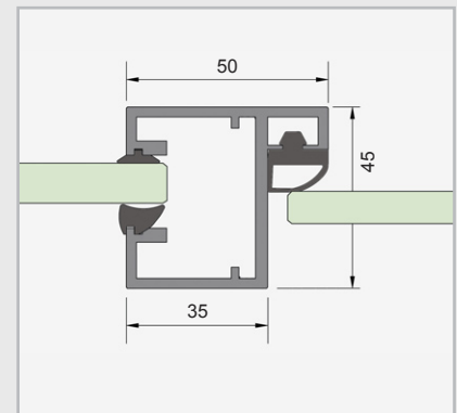
Profilé de dormant, raccord profilé mural
