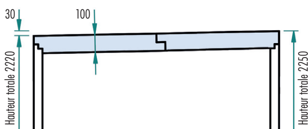
Forme de toit MONO
