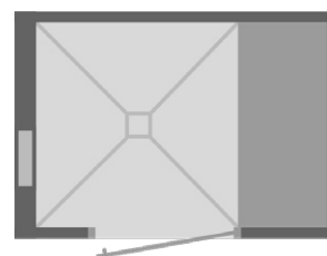
CAB-R 1780/1250 R.RL * Porte DIN droite / Banquette à droite de la porte / Panneau d'installation à gauche de la porte
