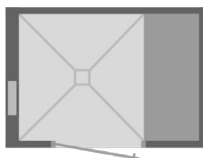
CAB-R 1780/1250 L.RL * Porte DIN gauche / Banquette à droite de la porte / Panneau d'installation à gauche de la porte
