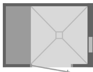
CAB-R 1780/1250 L.LR * Porte DIN gauche / Banquette à gauche de la porte / Panneau d'installation à droite de la porte
