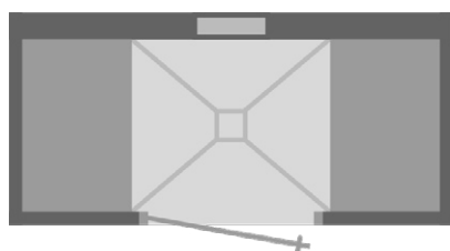
CAB-R 2000/950 L Porte DIN gauche / Banquette à gauche et à droite de la porte / Panneau d'installation à l'opposé de la porte
