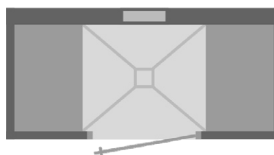
CAB-R 2000/950 R Porte DIN droite / Banquette à gauche et à droite de la porte / Panneau d'installation à l'opposé de la porte
