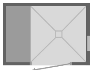
CAB-R 1780/1250 R.LR * Porte DIN droite / Banquette à gauche de la porte / Panneau d'installation à droite de la porte
