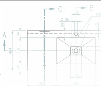
Waschtisch LAVADO PLUS Individuelle Sonderform → Seite 78
