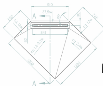
Duschboden mit Linienentwässerung TUB-LINE PLUS Individuelle Sonderform → ab Seite 34
