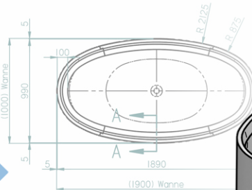
Wannenverkleidung TOP-TR PLUS Individuelle Sonderform → Seite 72
