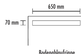
Bodenablaufrinne
