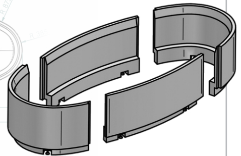
Wannenverkleidung TOP-TR PLUS Individuelle Sonderform → Seite 72
