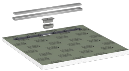
Duschboden mit Linienentwässerung TUB-LINE Standardprodukt
