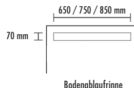
Bodenablaufrinne
