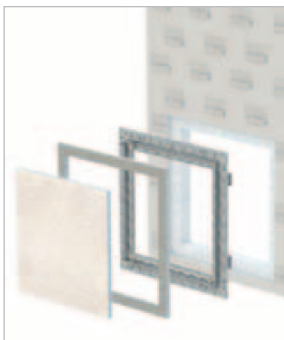
Anwendung bei Putz: mit Frontplatte / Füllstücke auf Rahmen
