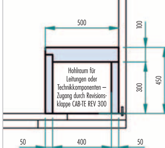
Maße Sitzbank
