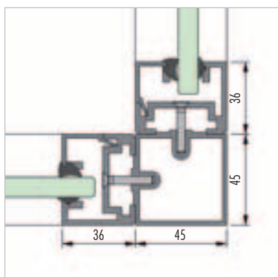
5 2x Wandprofil mit Eckprofil 90°
