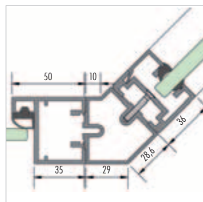
6 Zargenprofil mit Eckprofil 135° + Wandprofil
