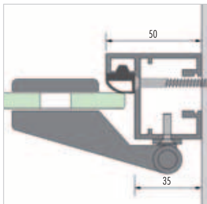
2 Zargenprofil Türband, Wandanschluss
