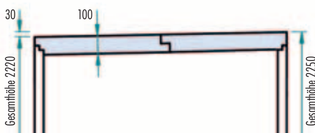
Dachform MONO
