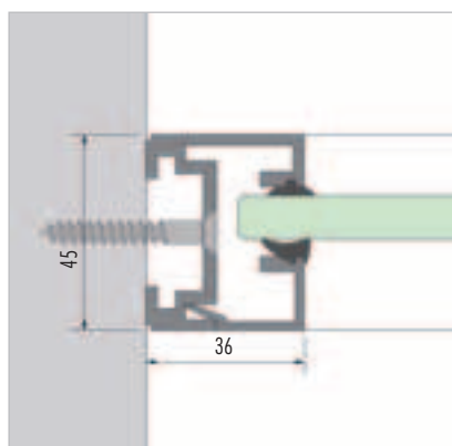
4 Wandprofil, Wandanschluss
