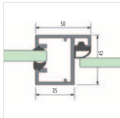
3 Zargenprofil, Anschluss Wandprofil
