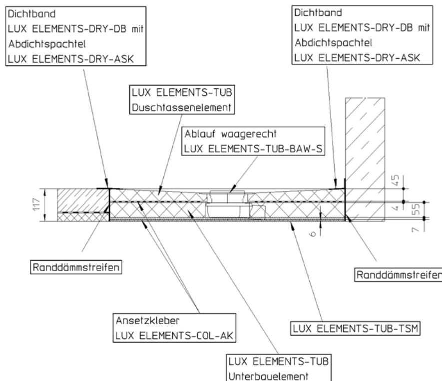
Abbildung 1: LUX ELEMENTS-TUB mit waagerechtem Ablauf und Unterbauelement
